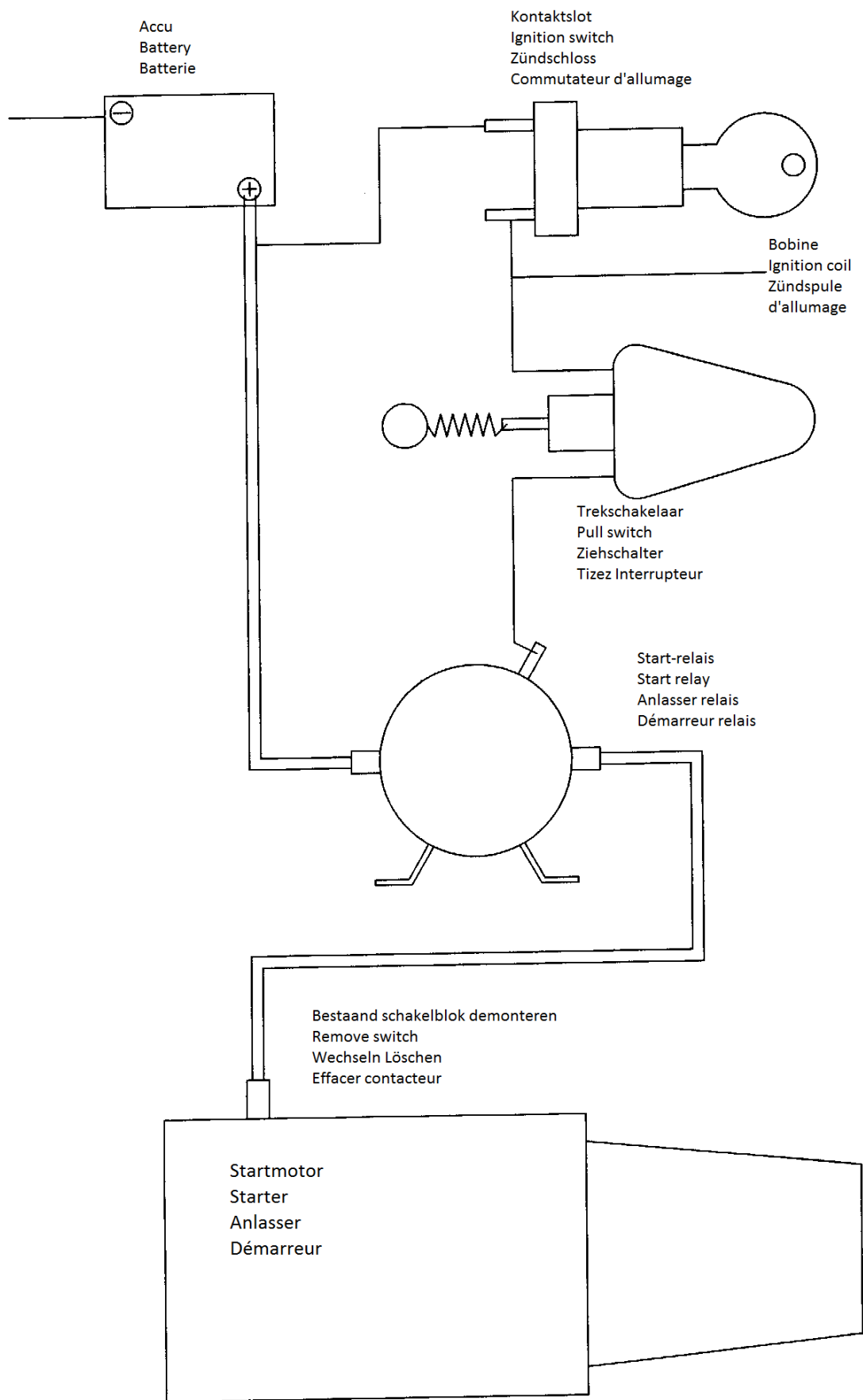
Aansluitschema startrelais Connection diagram Start relay Anschlussplan Anlasser relais Schéma de connexion Démarreur relais
