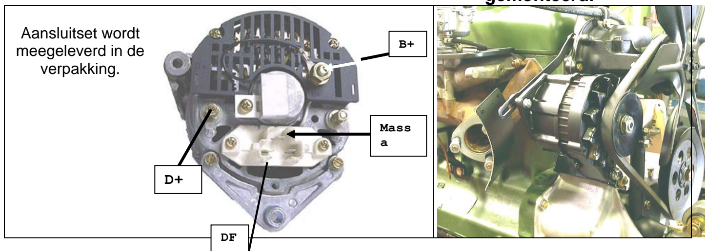
Dynamo op motor gemonteerd.
