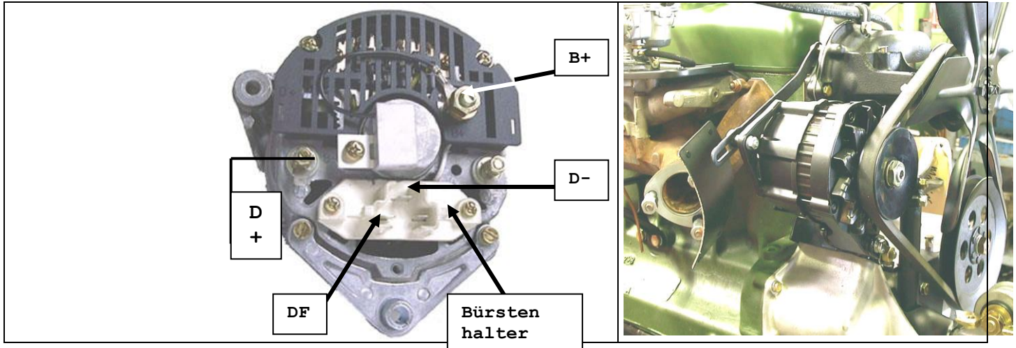
Generator Rückseite.
