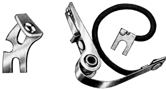
Contact jeu de rupteur Ducellier: art.nr. DM211-17
