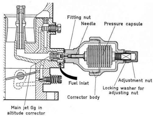
Fig. 41 SOLEX Altitude Corrector
